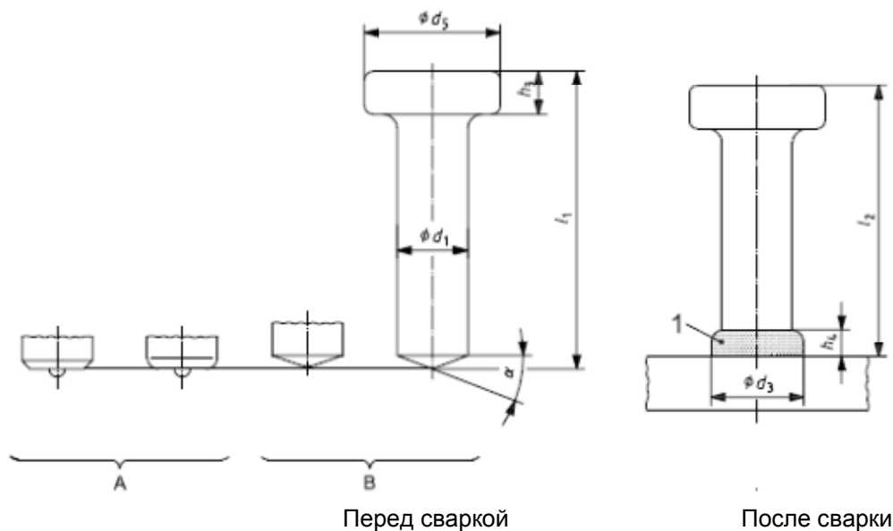
Рисунок 5 – Шпилька-упор (SD)
